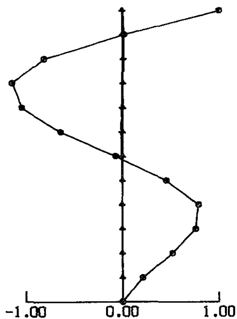
MODE 8
