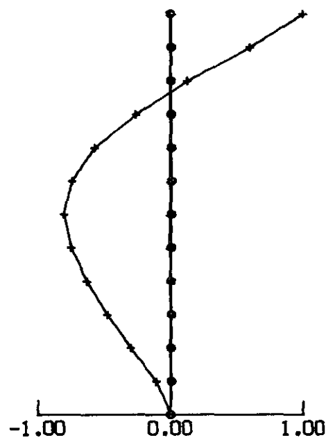
MODE 4 0.796 HZ.
