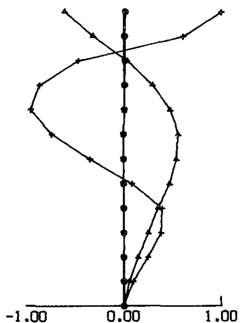
MODE 7
