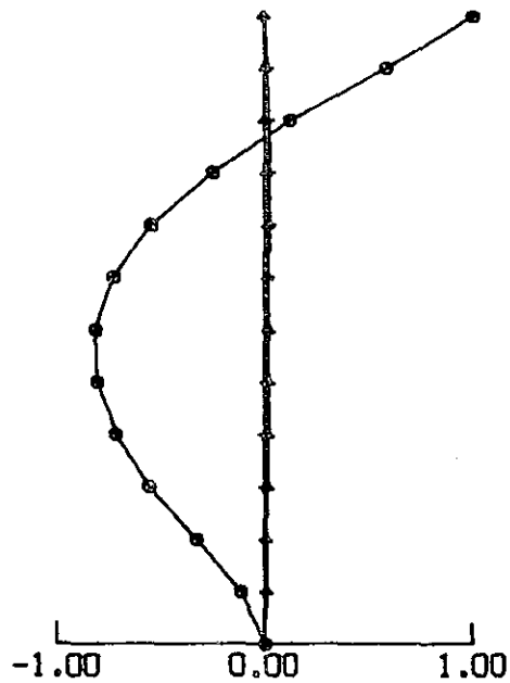
MODE 5
