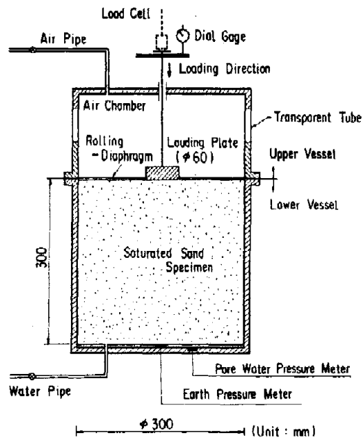
Fig. 18 Test Apparatus
