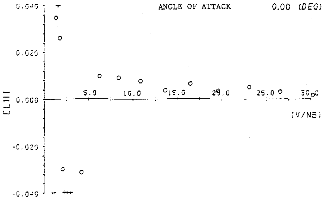
Fig. 4-2 C_{LH}^I - V/NB (Model No. 16)
